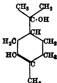
\alpha -Terpineol.
